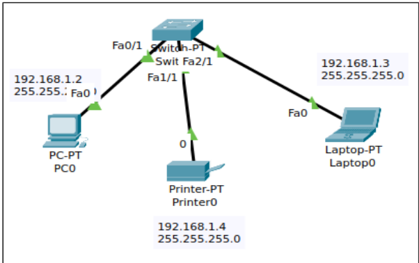
Figure 1. Réseau simple en Ethernet
